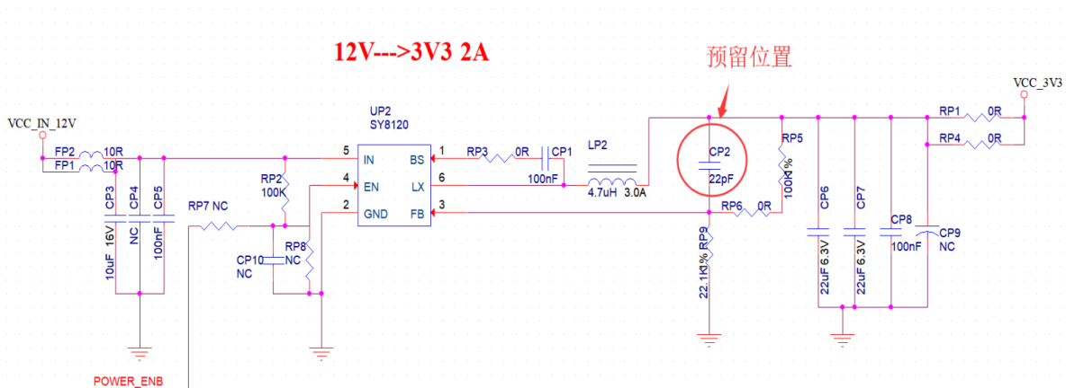
图 14 DC-DC 降压电路图
