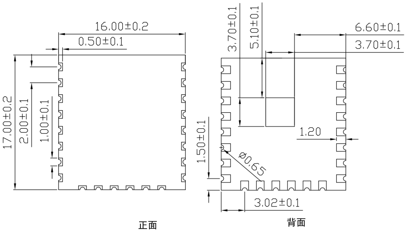
图 4 尺寸图
