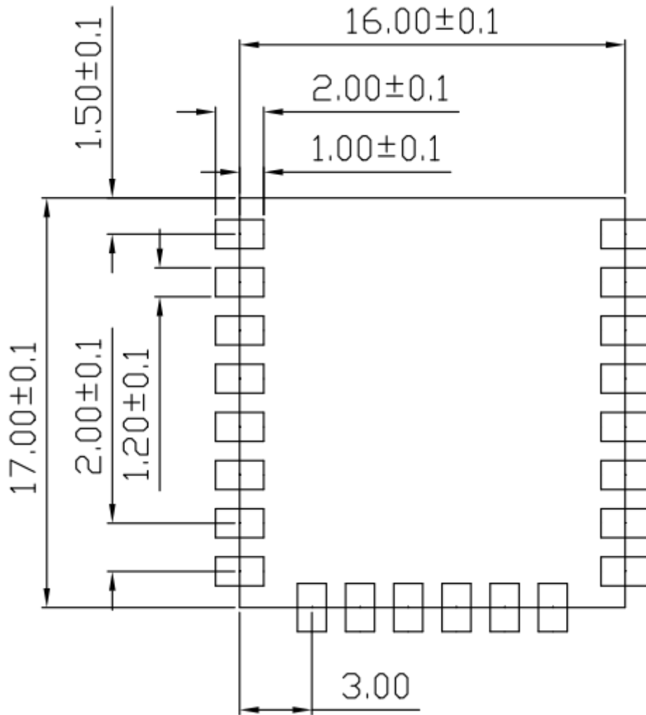
图 9 推荐 PCB 封装尺寸
