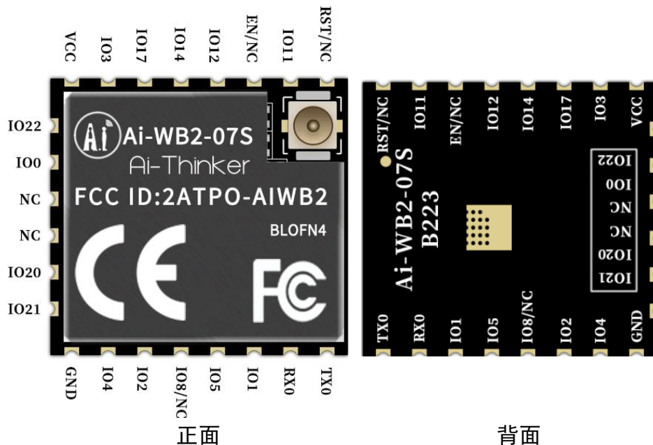
图 6 管脚示意图
